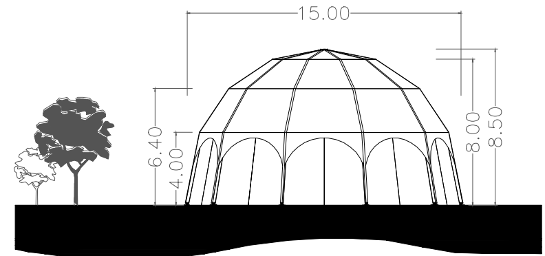
HAUPTANSICHT
