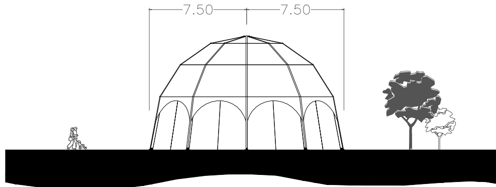
SEITENANSICHT
