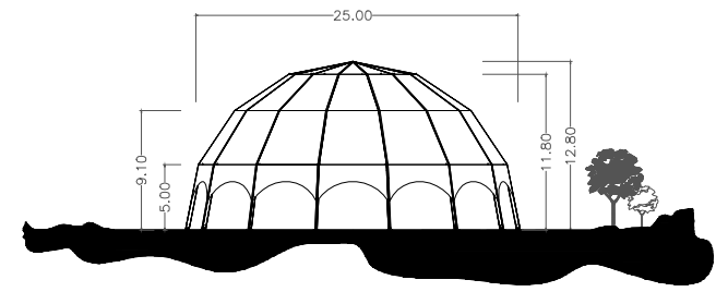
HAUPTANSICHT
