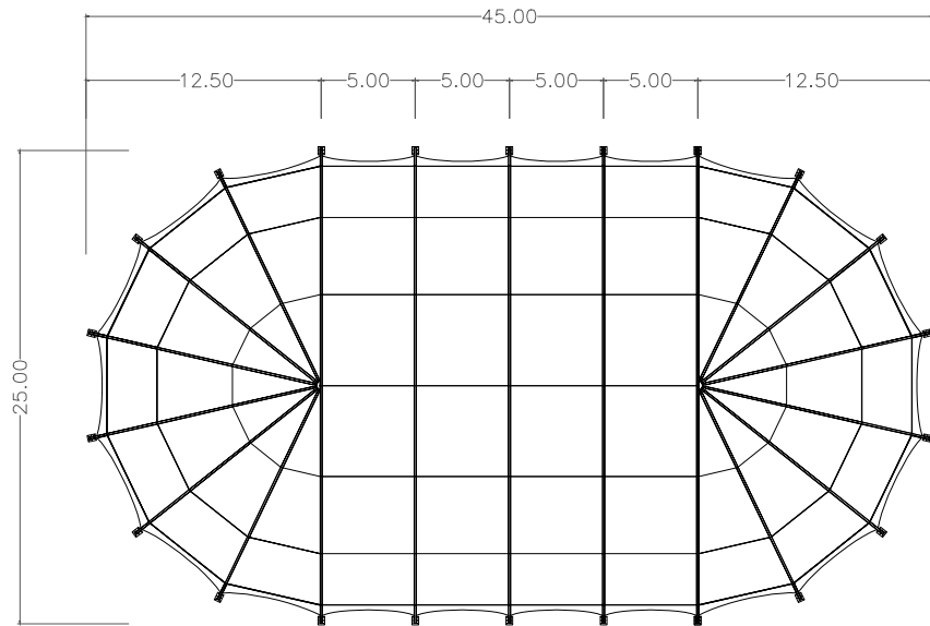
DRAUFSICHT
