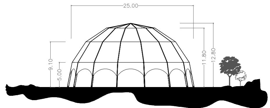
HAUPTANSICHT
