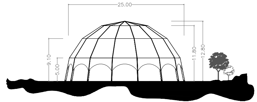
HAUPTANSICHT
