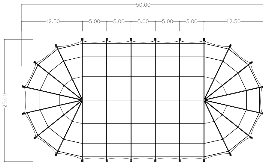
DRAUFSICHT
