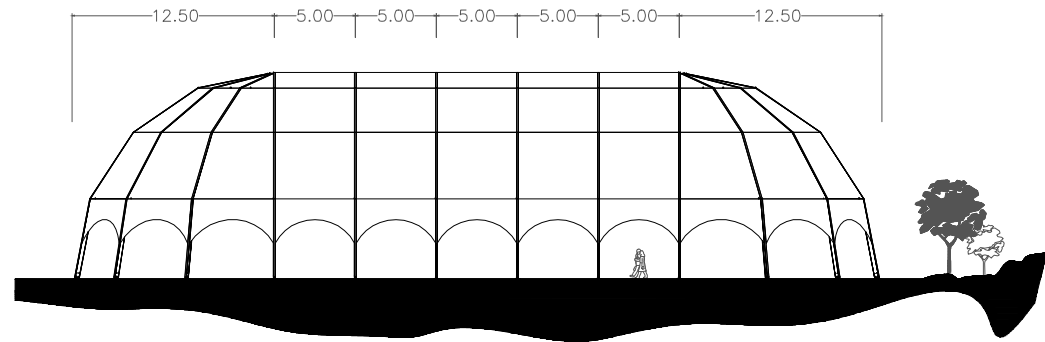
SEITENANSICHT
