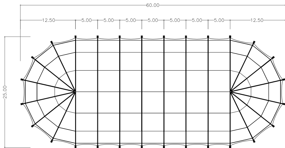
DRAUFSICHT
