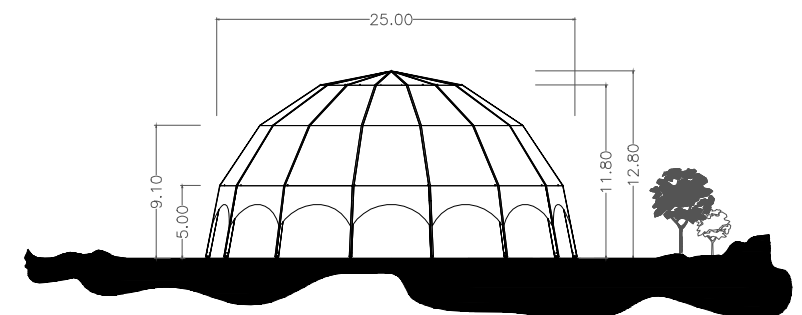
HAUPTANSICHT
