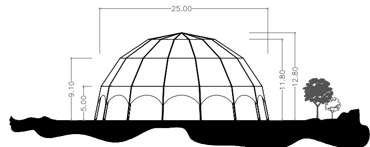
HAUPTANSICHT
