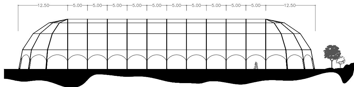
SEITENANSICHT
