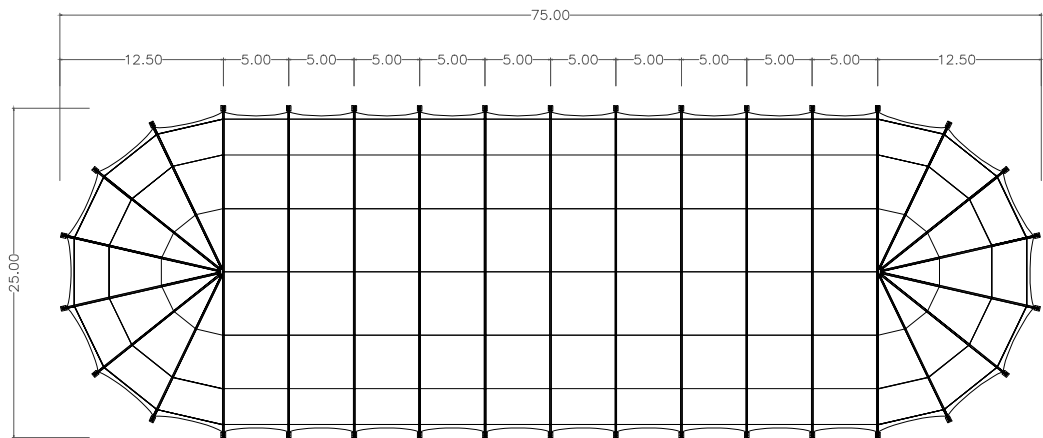
DRAUFSICHT
