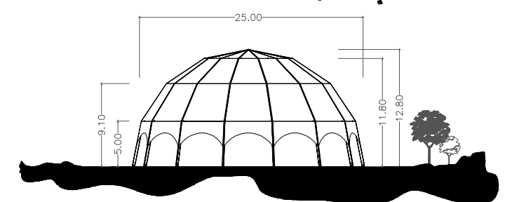
HAUPTANSICHT
