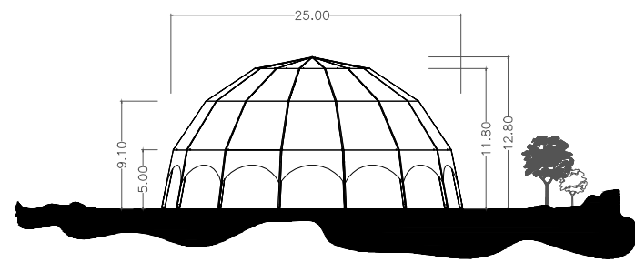
HAUPTANSICHT
