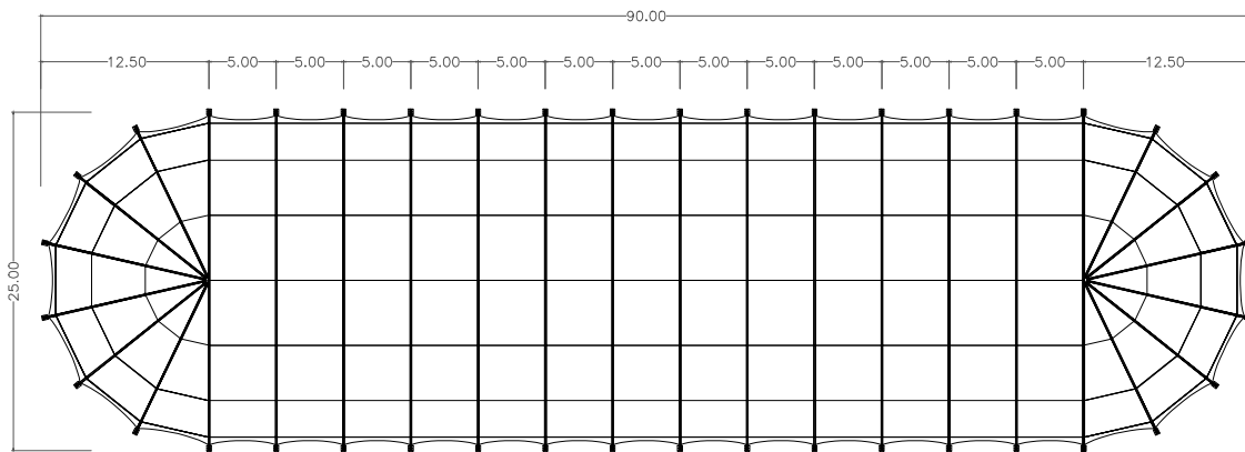
DRAUFSICHT
