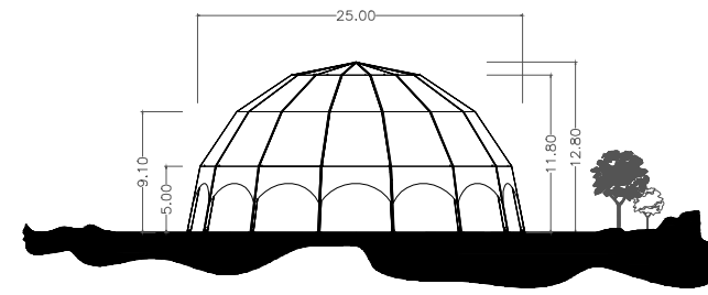
HAUPTANSICHT
