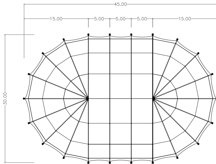
DRAUFSICHT
