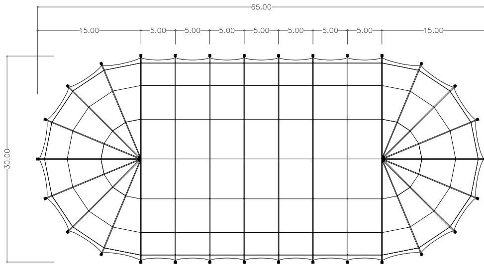
DRAUFSICHT
