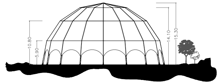
HAUPTANSICHT
