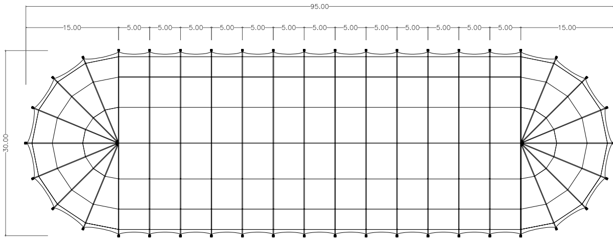
DRAUFSICHT
