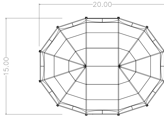
DRAUFSICHT
