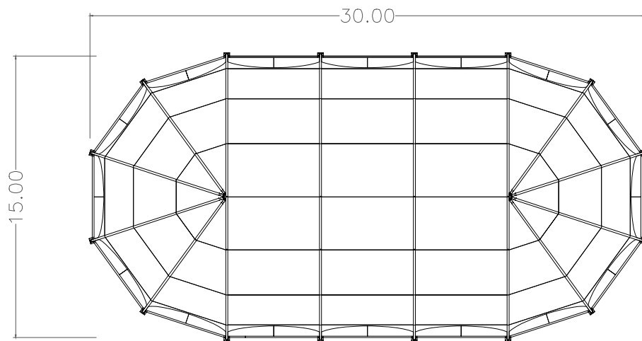
DRAUFSICHT
