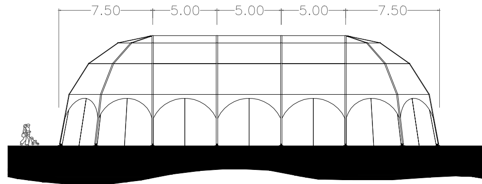
SEITENANSICHT
