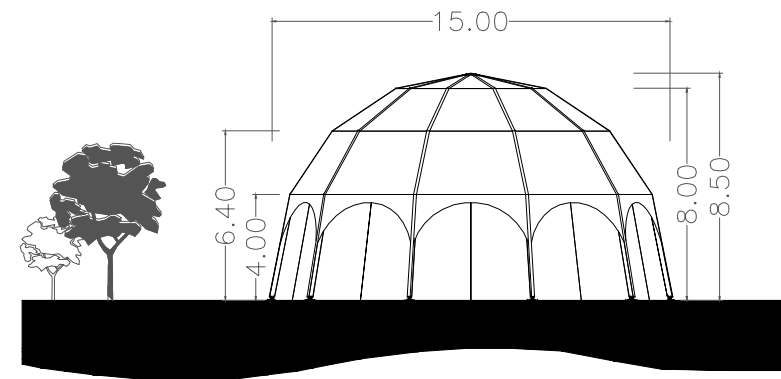
HAUPTANSICHT
