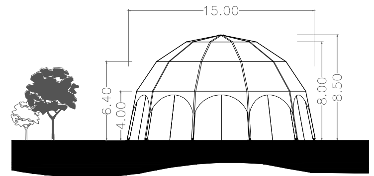
HAUPTANSICHT
