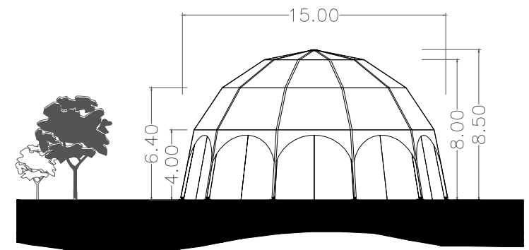
HAUPTANSICHT
