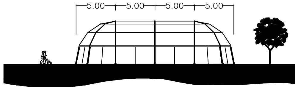
SEITENANSICHT
