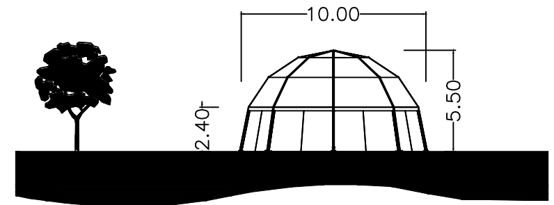
HAUPTANSICHT
