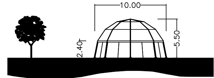
HAUPTANSICHT
