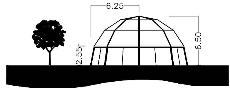
HAUPTANSICHT
