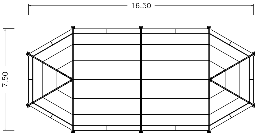
DRAUFSICHT
