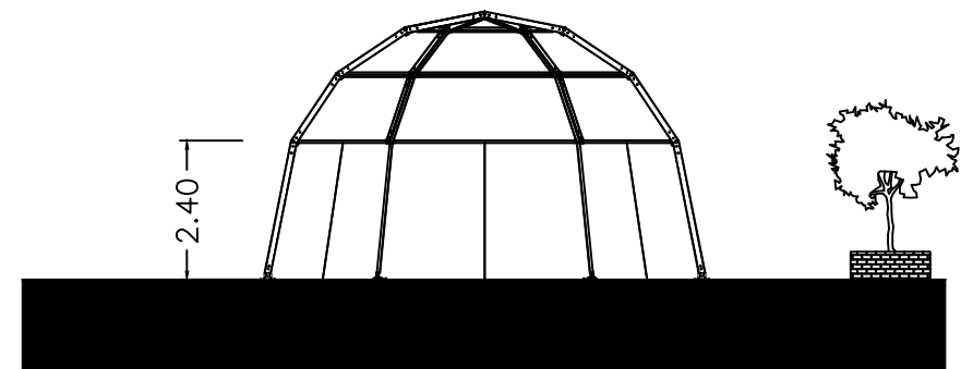
SCHNITT
