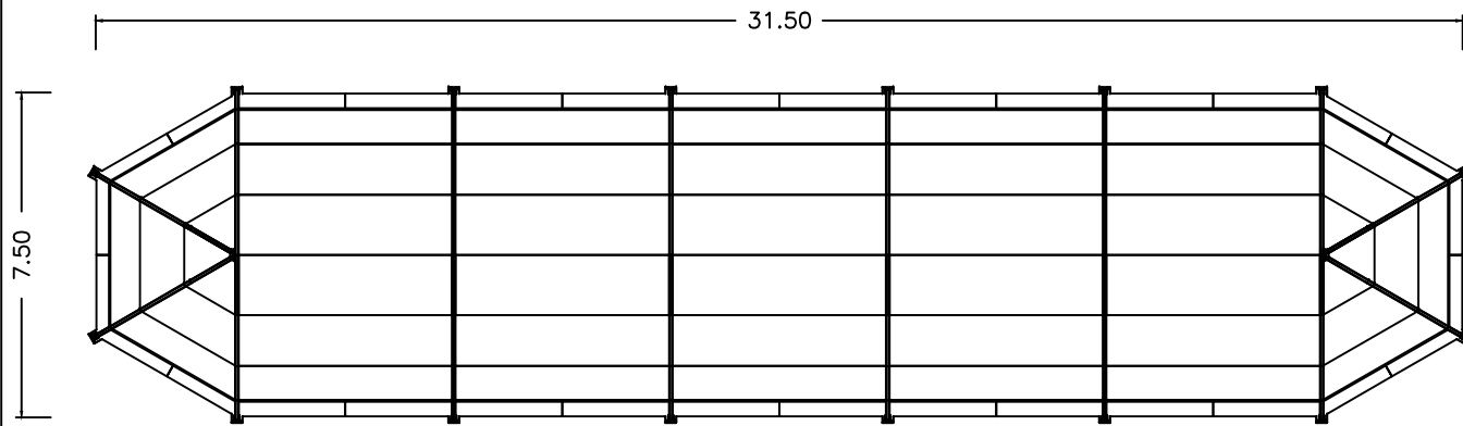
DRAUFSICHT
