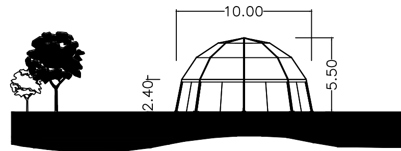
HAUPTANSICHT
